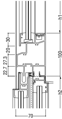
19 引違い / FIX
