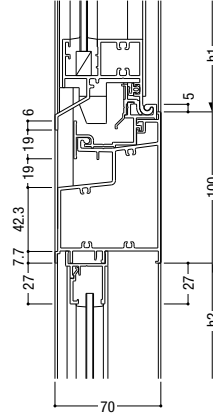
119 インベイ内倒し排煙 / FIX
