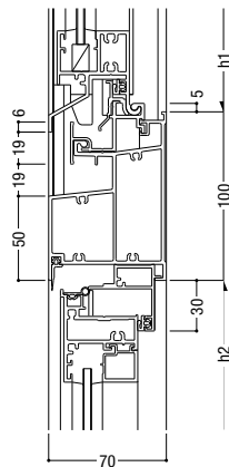
38 インペイ内倒し排煙 / 外開き・たてすべり
