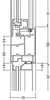
95 内倒し排煙 / FIX
