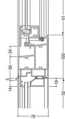
96 内倒し排煙 / FIX
