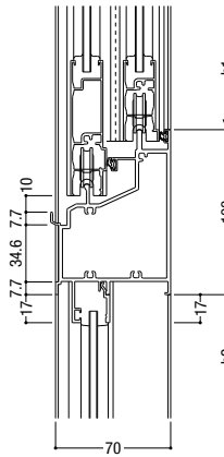
75 外動片引き / FIX
