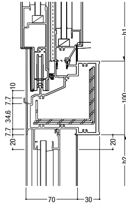
83 すべり出し・突出し / FIX
