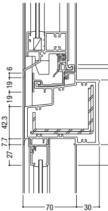
122 インベイ内倒し排煙 / FIX
