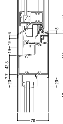
120 インベイ内倒し排煙 / FIX
