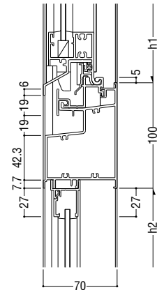
32 突出し排煙 (インペイと共通) / FIX
