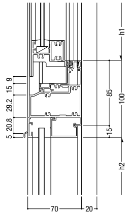
87 外倒し排煙(インペイト共通) / FIX
