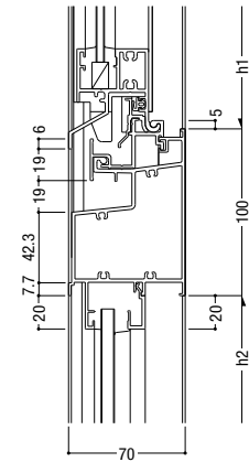
100 内倒し排煙 / FIX
