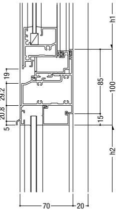
85 外倒し排煙(インペイト共通) / FIX
