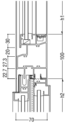
18 引違い / FIX
