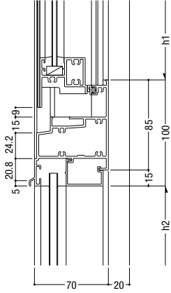
117 インベイ内倒し排煙 / FIX
