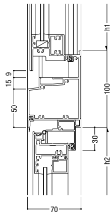
40 FIX / 外開き・たてすべり
