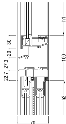
11 外動片引き / 外動片引き
