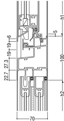
8 FIX / 引違い
