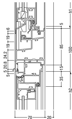
39 インペイ内倒し排煙 / 外開き・たてすべり
