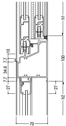
76 外動片引き / FIX
