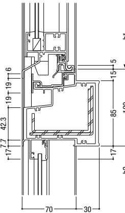
121 インベイ内倒し排煙 / FIX
