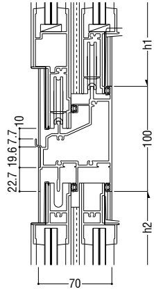
6 インペイ内倒し排煙 / 引違い
