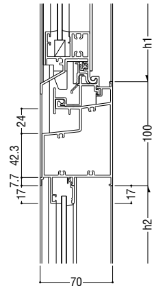
31 突出し排煙 (インペイと共通) / FIX
