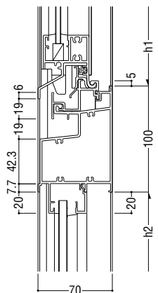
33 インペイ内倒し排煙 / FIX
