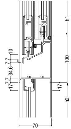
20 外動片引き / FIX
