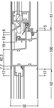
98 内倒し排煙 / FIX
