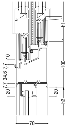
22 外動片引き / FIX
