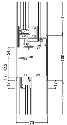
88 外倒し排煙(インペイト共通) / FIX
