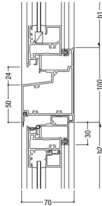
34 内倒し排煙 / 外開き・たてすべり
