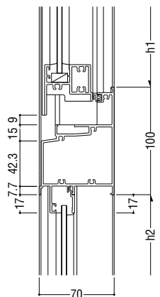
34 インペイ内倒し排煙 / FIX
