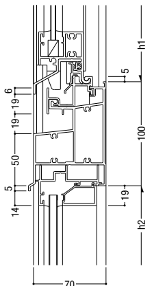
106 突出し排煙 (インペイト共通) / FIX
