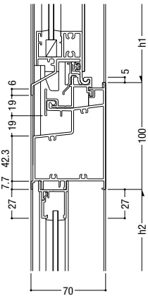
99 内倒し排煙 / FIX
