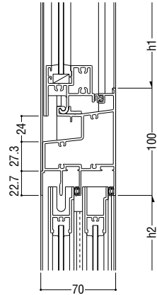
7 FIX / 引違い
