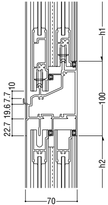
5 突出し排煙 (インペイと共通) / 引違い
