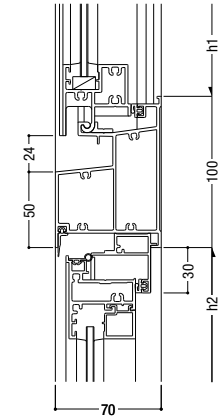
36 突出し排煙 (インペイと共通) / 外開き・たてすべり
