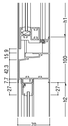
35 インペイ内倒し排煙 / FIX
