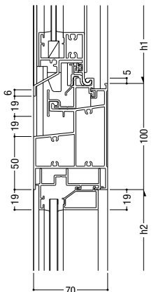
105 突出し排煙 (インペイト共通) / FIX
