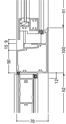
72 引違い / FIX
