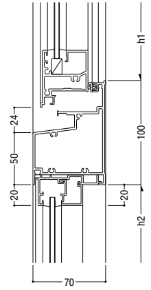
84 外倒し排煙(インペイト共通) / FIX
