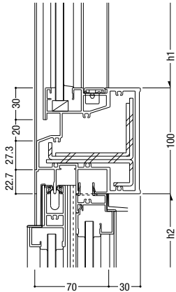
33 外倒し排煙 (インペイと共通) / 外開き・たてすべり
