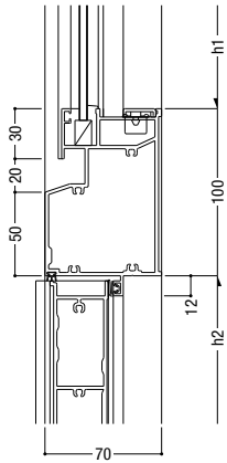
74 外動片引き / FIX
