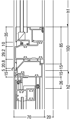
69 インペイ内倒し排煙 / 片開きドア・両開きドア
