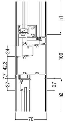
29 内倒し排煙 / FIX
