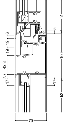
118 インベイ内倒し排煙 / FIX
