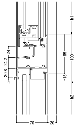
97 内倒し排煙 / FIX
