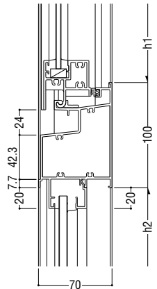
30 突出し排煙 (インペイと共通) / FIX
