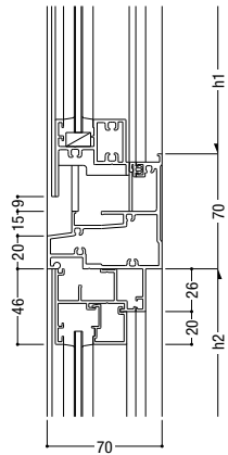
86 外倒し排煙(インペイト共通) / FIX
