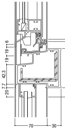
123 インベイ内倒し排煙 / FIX
