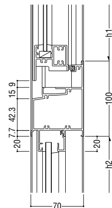
36 FIX / FIX
